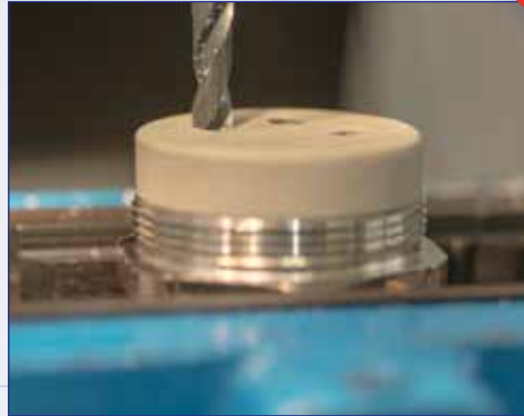
Bohren von Dichteinsätzen für Kabelverschraubungen Drilling of inserts for cable glands Perforation d'inserts pour presse-étoupes
