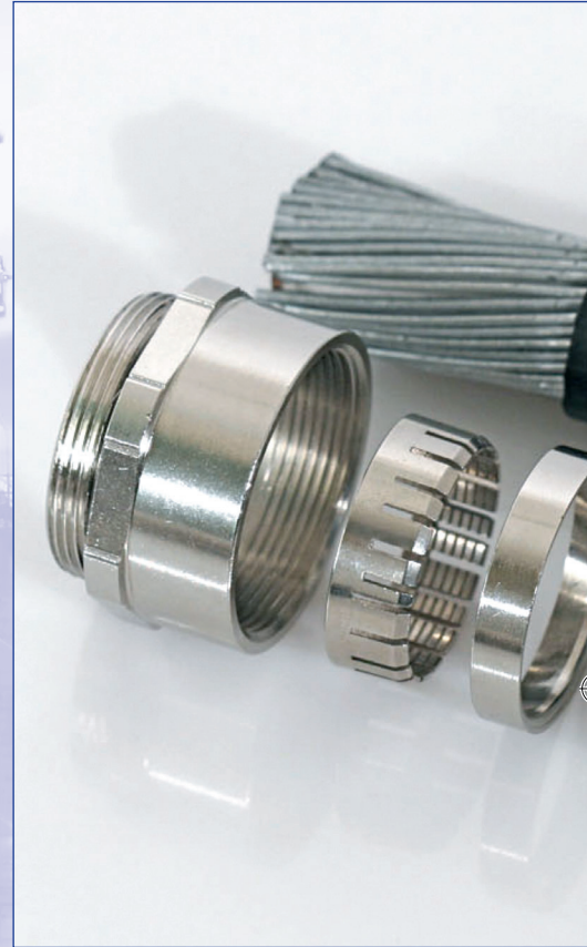
Pflitsch Exe blueglobe AC armierte Kabel Pflitsch Exe blueglobe AC armoured cable Pflitsch Exe blueglobe AC câble armé
