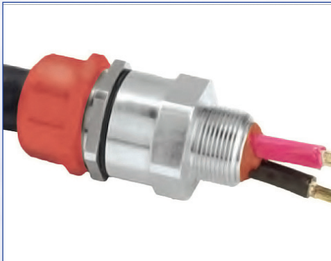
CMP Exd Kabelverschraubung mit Vergussmasse CMP Exd barrier gland CMP Exd avec résine
